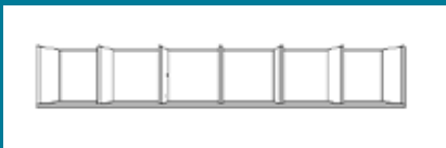
01 1 single module H/W/D 32,1/193,8/30,5 cm 01 1 enkelt modul H/B/D 32,1/193,8/30,5 cm
