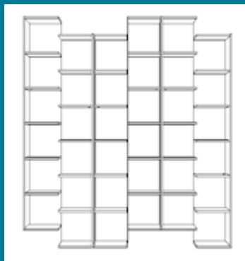
06 2 single modules and 2 double modules H/W/D 217,8/189,2/30,5 cm 06 2 enkelte moduler og 2 dobbelte moduler H/B/D 217,8/189,2/30,5 cm
