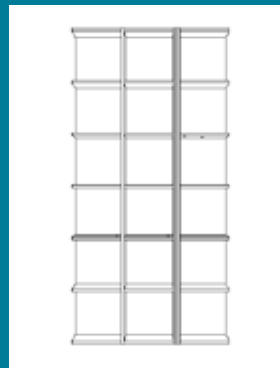
03 1 double module and 1 single module H/W/D 193,8/94,6/30,5 cm 03 1 dobbelt modul og 1 enkelt modul H/B/D 193,8/94,6/30,5 cm
